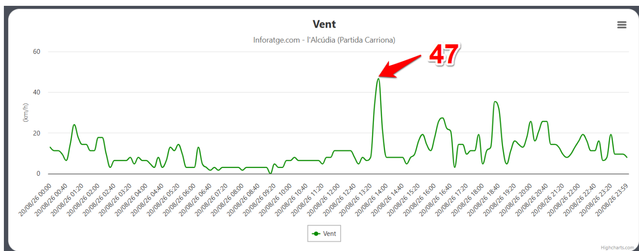
Ráfagas de viento máximas registradas en l'ALCÚDIA (estación Partida Carriona) el 20/08/26 (en km/h) https://inforatge.com/meteo-lalcudia
