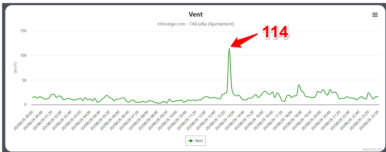
Ráfagas de viento máximas registradas en l'ALCÚDIA (núcleo urbano) el 20/08/26 (en km/h) https://inforatge.com/meteo-lalcudia
