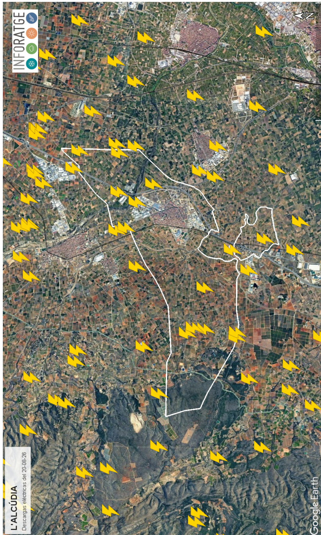
Geolocalización de las descargas eléctricas nube-tierra registradas en el término municipal de L' ALCÚDIA y alrededores el 20/08/2018 Fuente descargas: AEMET Agencia Estatal de Meteorología // Cartografía: © Instituto Geográfico Nacional de España
